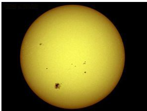
Diámetro del Sol: 1.392.000 km.
